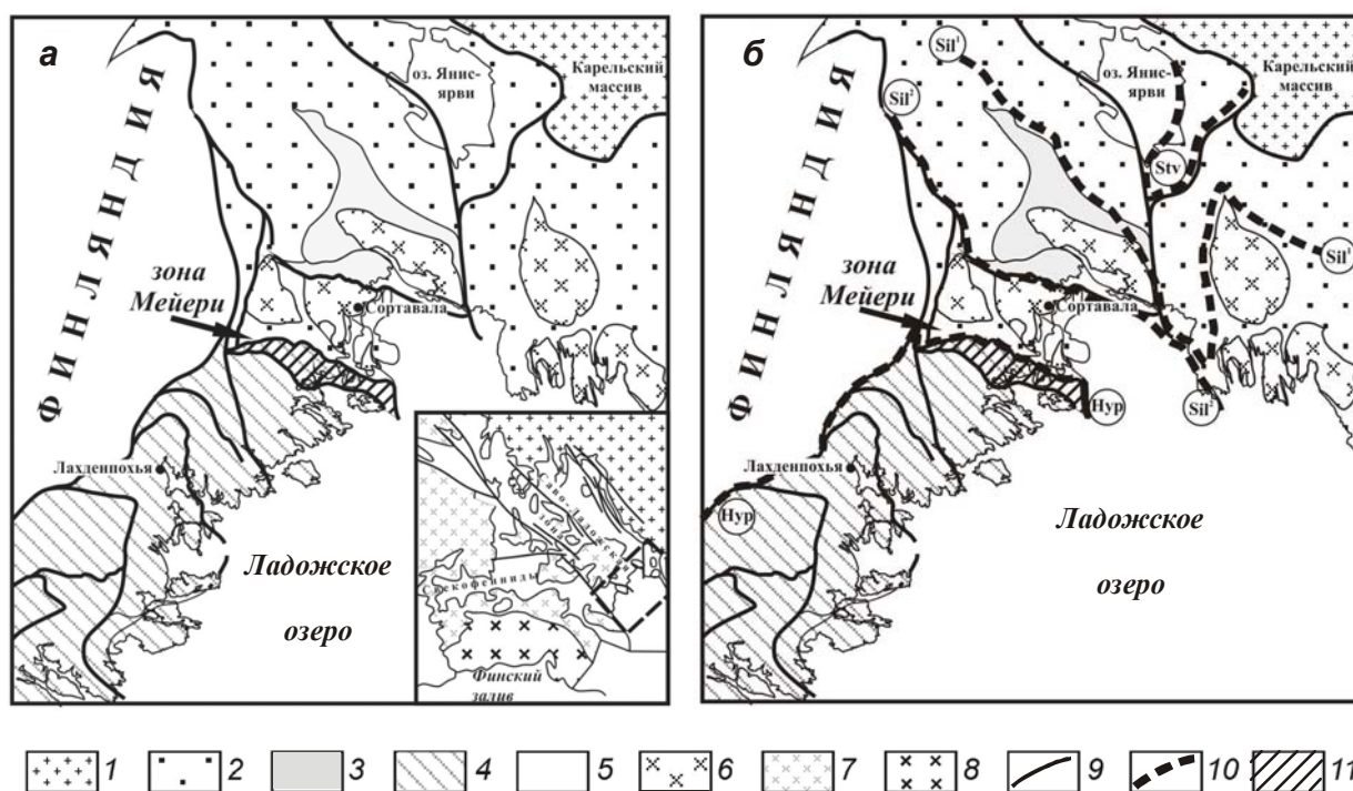
Рис. 1. Схемы геологического строения (а) и метаморфизма (б) изученного района. На врезке – его положение в Свекоскарельской подвижной области
