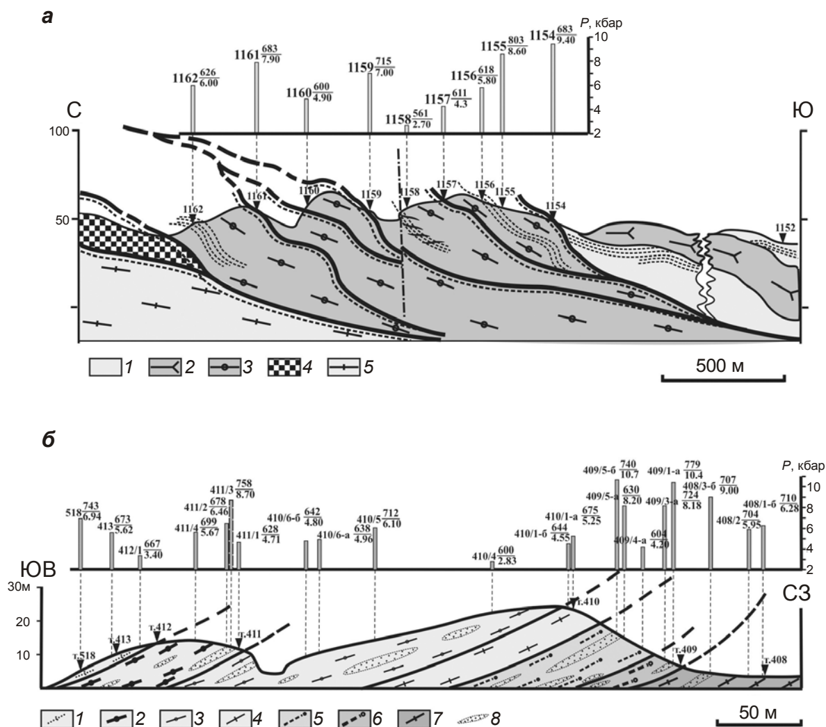
Рис. 11. Профили через зону Мейери в районе оз. Куоккаярви (а) и о. Хавус (б) в сопоставлении с рассчитанными значениями PT -параметров
