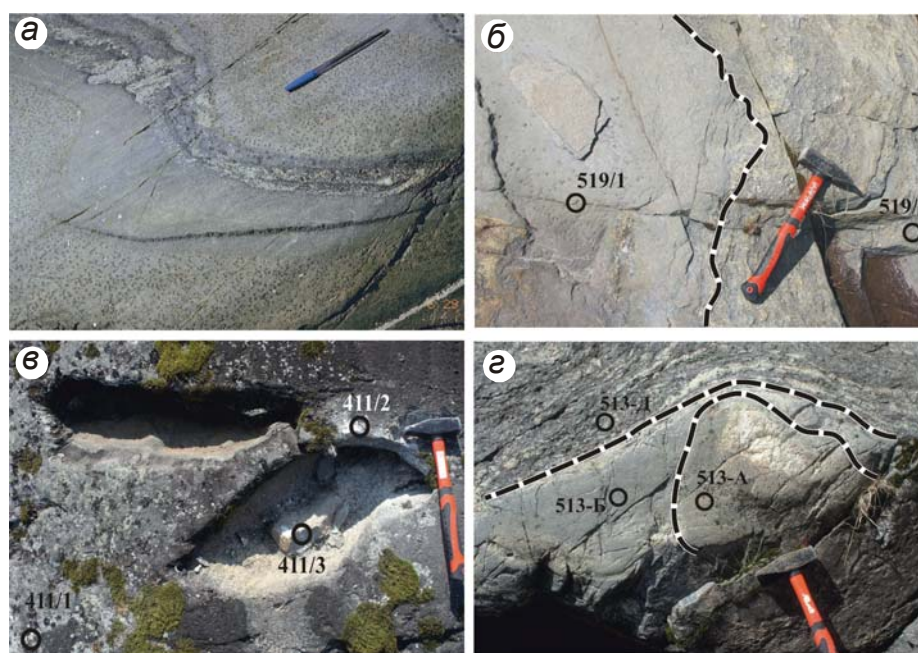
Рис. 12. Неоднородность распределения тектонитов в дециметровом диапазоне (о. Хавус)
