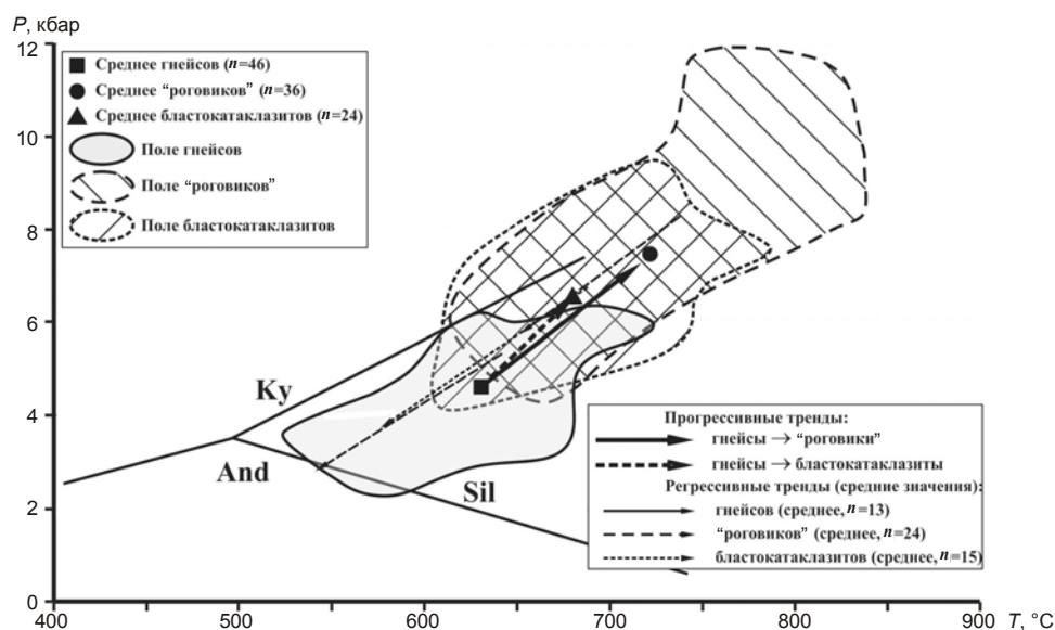
Рис. 15. Тренды стресс-метаморфизма двух стадий (ороговикования и бластокатаклаза), рассчитанные по средним значениям P - T -параметров для регионально метаморфизованных пород «матрицы» тектонитов, «роговиков» и бластокатаклазитов. n — число анализов по группам пород)
