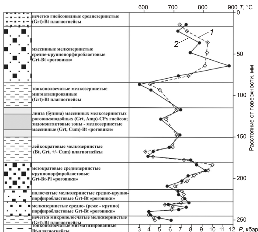
Рис. 13. Неоднородность распределения тектонитов, слабо тектонизированных и нетектонизированных гнейсов/плаггио-гнейсов в субгоризонтальной тектонической пластине о. Хавус (по керну скважин) в сантиметровом диапазоне
