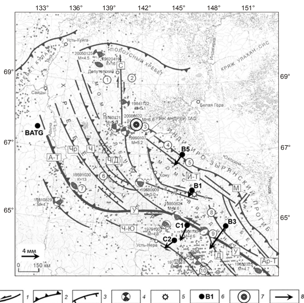
Рис. 4. Векторы скоростей горизонтальных смещений относительно пункта BATG (сейсмостектоника зоны хребта Черского приводится по [Имаев и др., 2009; Имаева, Козьмин, Имаев, 2009])
