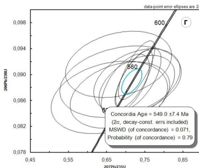
Рис. 7. Цирконовая проба 124-1. а, б – микроскопические фотографии порфиробластовых эпидотовых гнейсов в скрещенных николях; в – CL-фотографии цирконов пробы; г – конкордия.
