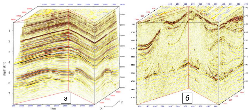
Рисунок 5. Примеры результатов COV-миграции с сохранением амплитуд: а) многолучевая асимптотическая миграция, Тимано-Печора; б) волновая псевдоспектральная миграция; Астраханский свод.
