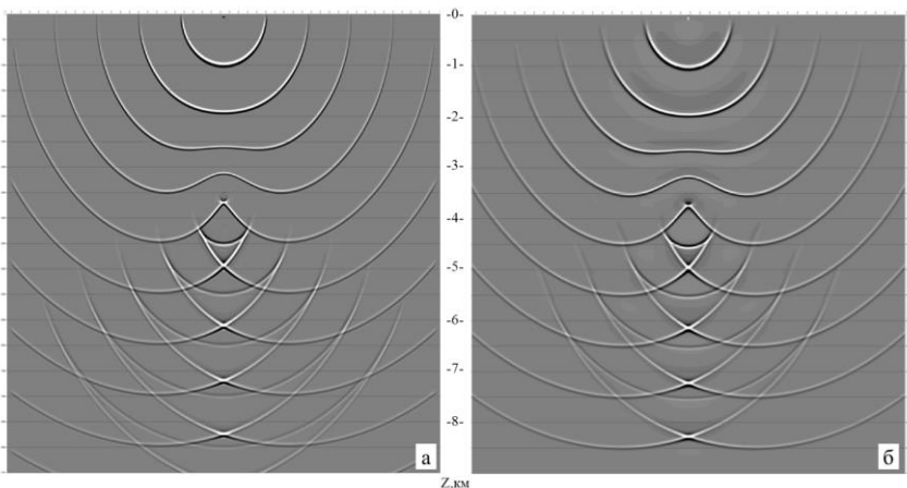
Рисунок 2. Сравнение результатов расчета волн от точечного источника для 3-D модели среды с низкоскоростным включением: а) конечно-разностное решение волнового уравнения; шаг пространственной сетки расчета 2,5м; б) псевдоспектральное решение одностороннего волнового уравнения; шаг пространственной сетки расчета 25м.
