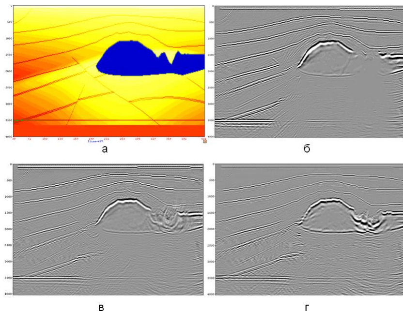
Рисунок 3. Сравнение разрезов XL 437 различных 3-D глубинных миграций до суммирования на синтетических данных SEG Salt: а) вертикальное сечение модели; б) однолучевая миграция Кирхгофа с «лучевыми» весами; в) многолучевая; г) псевдоспектральная.
