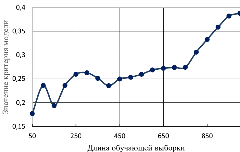
Рисунок 6. Зависимость качества модели от длины обучающей выборки
