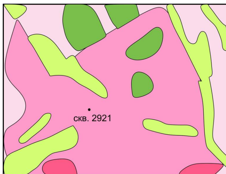
Рисунок 3. Фрагмент геологической карты курского блока ВКМ: 1 – обоянская серия (AR1ob); 2 – александровская свита (AR2al); 3 – плагиограниты салтыковского комплекса (рγAR2sl); 4 – щелочные граниты атаманского комплекса (δγAR2a); 5 – габброиды смородинского комплекса
