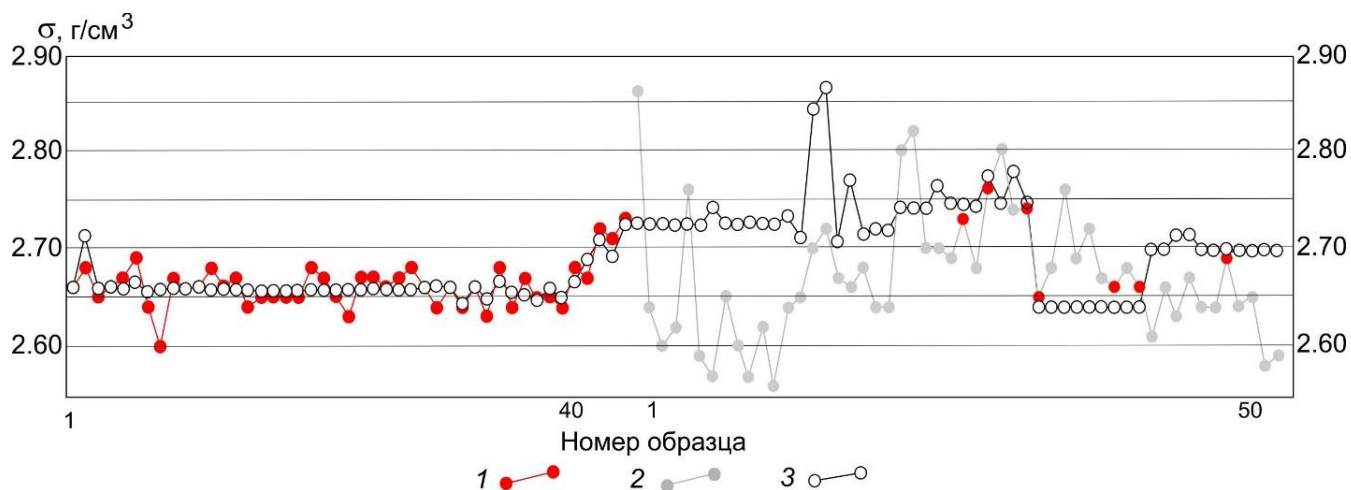
Рисунок 2. Идентификация мигматитов нерасчлененной михайловской серии: 1 – экспериментальные значения плотности мигматитов александровской свиты; 2 – экспериментальные значения плотности мигматитов нерасчлененной михайловской серии; 3 – модельные значения плотности
