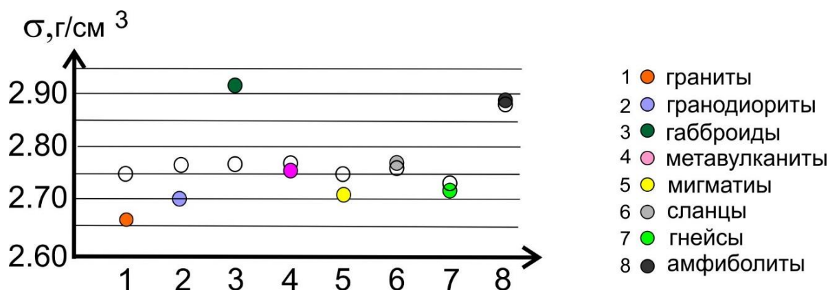
Рисунок 5. Экспериментальные (цветные кружки) и модельные (незакрашенные кружки) средних значений плотности основных литологических типов кристаллических пород ВКМ
