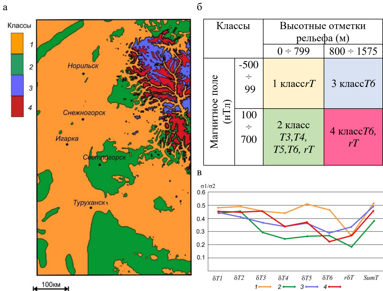
Рисунок 9. Результаты идентификационного моделирования: а – пространственная типизация площади исследования по значению комплексного признака; б – таблица реклассификации аномального магнитного поля и высотных отметок рельефа; в – средние значения \sigma_1/\sigma_2 для моделей, полученных для IMF - составляющих магнитного поля в пределах выделенных классов в соответствии с таблицей: 1 – класс 1; 2 – класс 2; 3 – класс 3; 4 – класс 4
