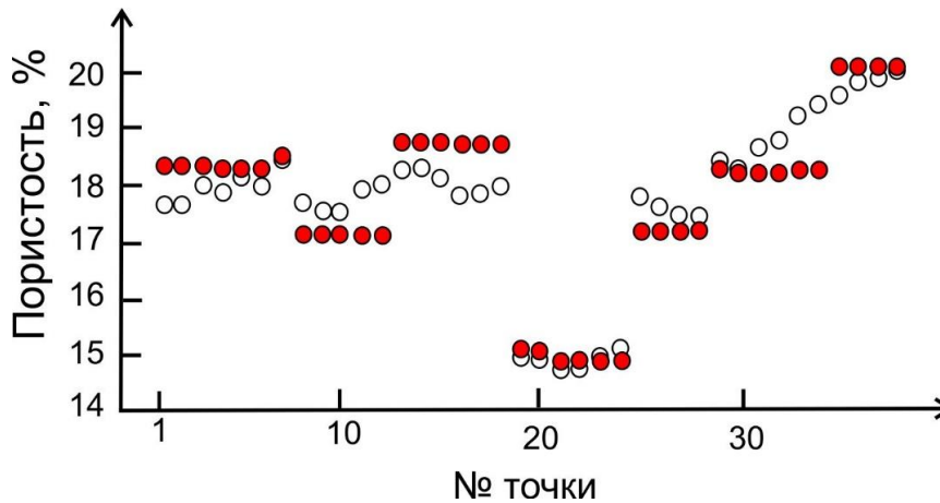
Рисунок 8. Соответствие фактических и модельных значений коэффициента пористости: красные кружки соответствуют экспериментальным значениям пористости; незаполненные – модельным значениям пористости
