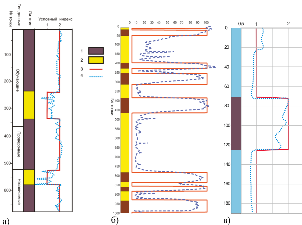
Рисунок 7. Результаты идентификационного моделирования по данным каротажа: а - идентификация коллектора среди вмещающих пород; б - выделение коллектора с использованием независимых данных по соседней скважине; в - определение типа коллектора. 1 – интервал коллектора; 2 – вмещающие породы; 3 – экспериментальные значения идентификатора коллектора; 4 – модельные значения идентификатора коллектора
