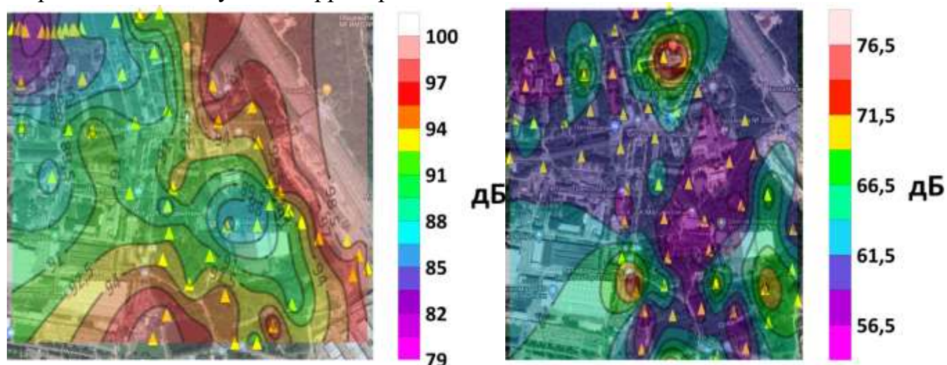
Рис. 16. Сопоставление карт распределения вибромикросейсмического (слева) и акустического (справа) загрязнения пос. Мосрентген, г. Москва
