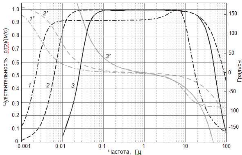
Рис. 8. Амплитудно-частотная (АЧХ) (1'–3') и фазо-частотная (ФЧХ) (1'–3') характеристики приборов Streckeisen (1, 1'), Guralp (2, 2') и СМЕ (3, 3')
