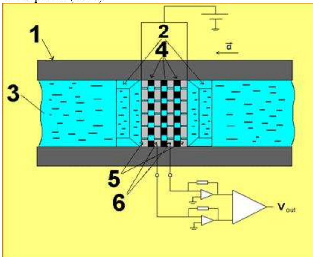
Рис. 5. Молекулярно-электронный преобразователь: 1 – диэлектрическая трубка (корпус преобразователя); 2,4 – установочные элементы; 3 – электролит; 5,6 – электроды
