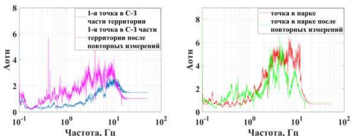
Рис. 17. Отношения спектральных амплитуд измерительный/опорный пункт: слева – в самой первой точке в лесопарковой зоне, вблизи промышленного предприятия (синяя кривая – первичные измерения, фиолетовая – повторные измерения), справа – в одной из точек в парке развлечений и отдыха (красная кривая – первичные измерения, зелёная – повторные измерения)
