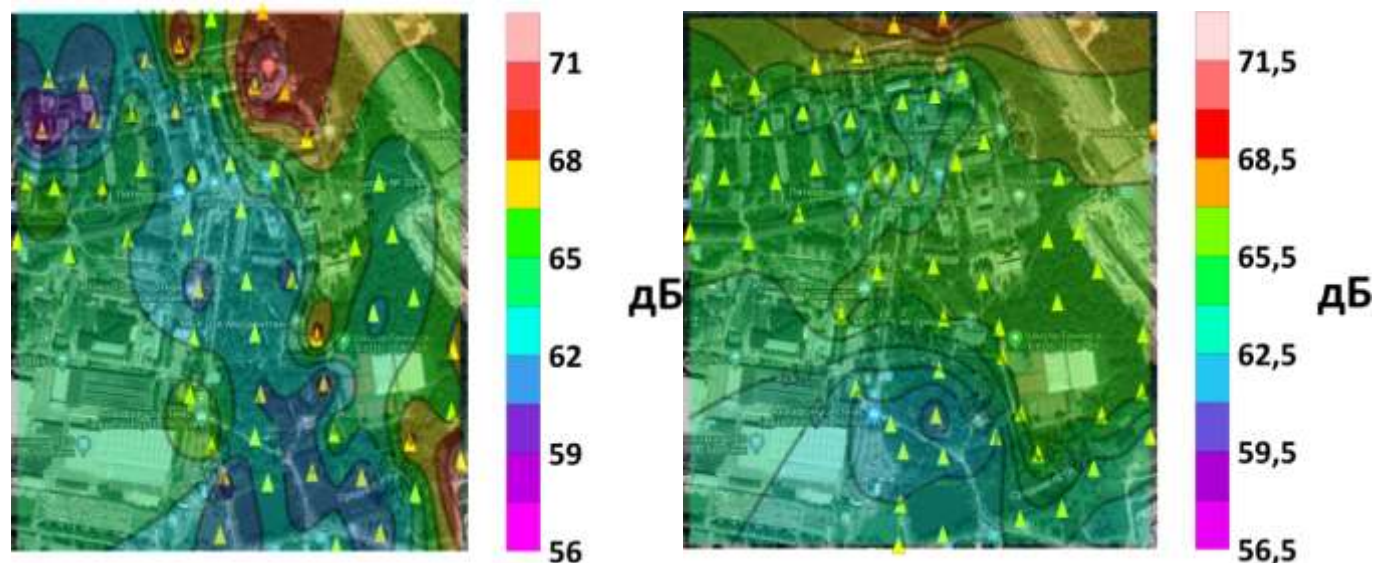
Рис. 14. Карты распределения уровней акустического шума на территории пос. Мосрентген для частоты 16 Гц: слева – день, справа – ночь
