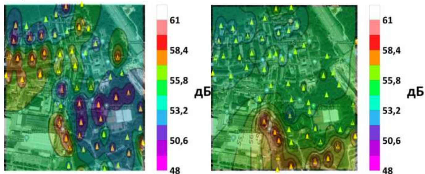
Рис. 15. Карты распределения уровней акустического шума на территории пос. Мосрентген для частоты 500 Гц: слева – день, справа – ночь
