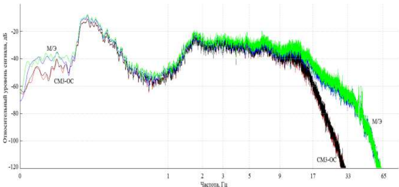
Рис. 7. Сравнение спектров двадцатиминутной синхронной записи двумя сейсмометрами СМЗ-ОС (чёрная и красная кривые) и двумя молекулярно-электронными сейсмометрами (синяя и зелёная кривые)
