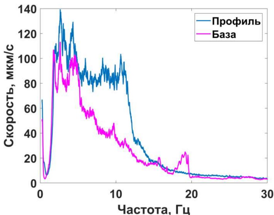
Рис. 10. Спектры записей с переносной и базовой станций
