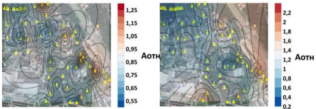
Рис. 3. Карты распределения относительных интенсивностей сейсмического поля на территории пос. Мосрентген для нескольких частот: слева – для частоты 4 Гц, справа – для частоты 8 Гц
