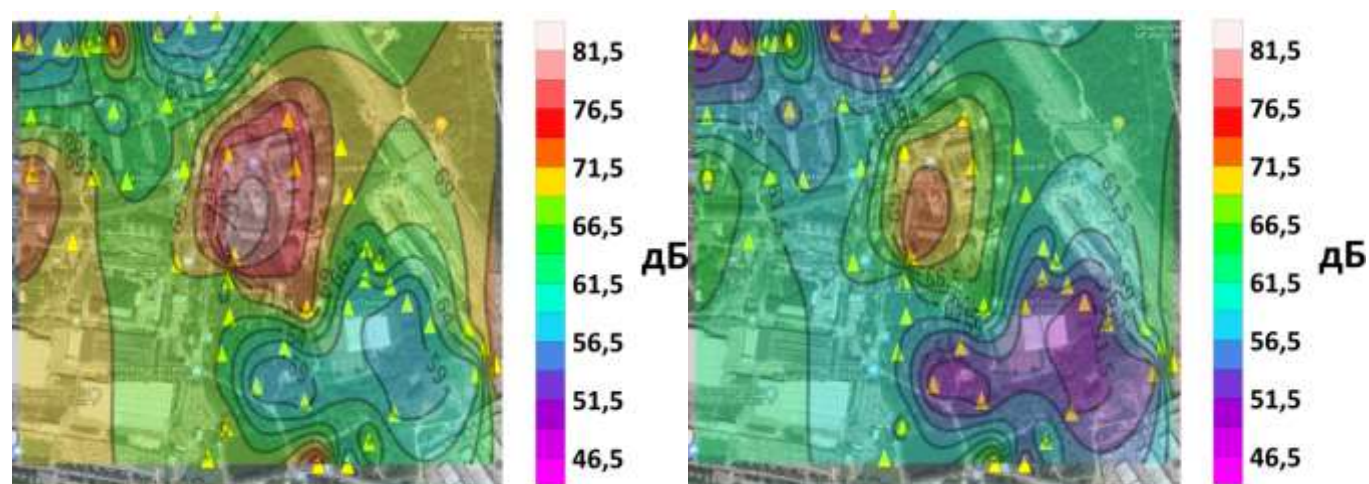
Рис. 13. Карты распределения вибромикросейсмического загрязнения на территории пос. Мосрентген для частоты 31,5 Гц: слева – день, справа – ночь. Уровень вибросейсмического фона в дневное время суток превышает аналогичный параметр за ночной период примерно на 8 дБ. Наиболее шумной является область, охватывающая центральную площадь пос. Мосрентген и близлежащие дворы – 71,5 – 79 дБ днём и 66,5 – 69 дБ ночью. Также относительно шумной является жилая
