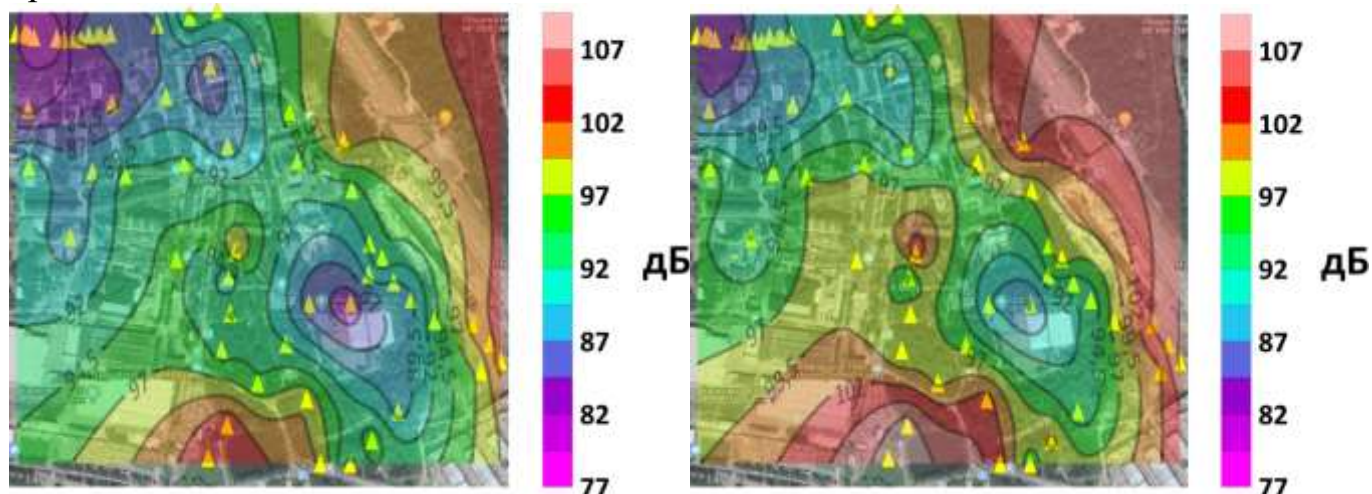
Рис. 12. Карты распределения вибромикросейсмического загрязнения на территории пос. Мосрентген для частоты 10 Гц: слева – день, справа – ночь. Уровень шума в ночное время суток выше, чем в дневное примерно на 3-5 дБ. Наиболее высокий уровень вибромикросейсмического загрязнения зафиксирован вблизи участка автострады МКАД-ЮГ, а также рядом с водоёмом у Проектируемого проезда № 139 и составляет около 99-102 дБ в дневное время суток и 102-105 дБ в ночное.
