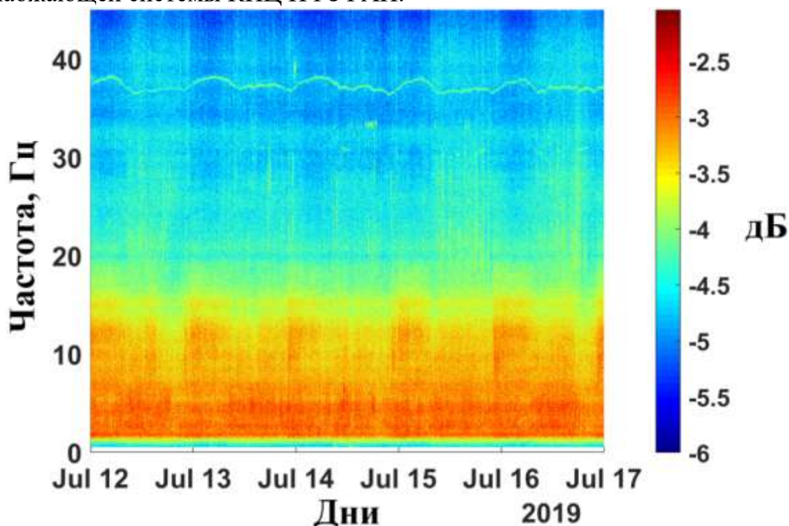
Рис. 11 Спектрограмма сигнала с опорного пункта в период с 12.07.2019 по 17.07.2019
