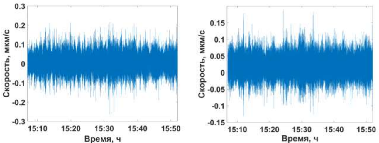
Рис. 9. Примеры записей волновых форм с переносной (слева) и базовой (справа) сейсмостанций
