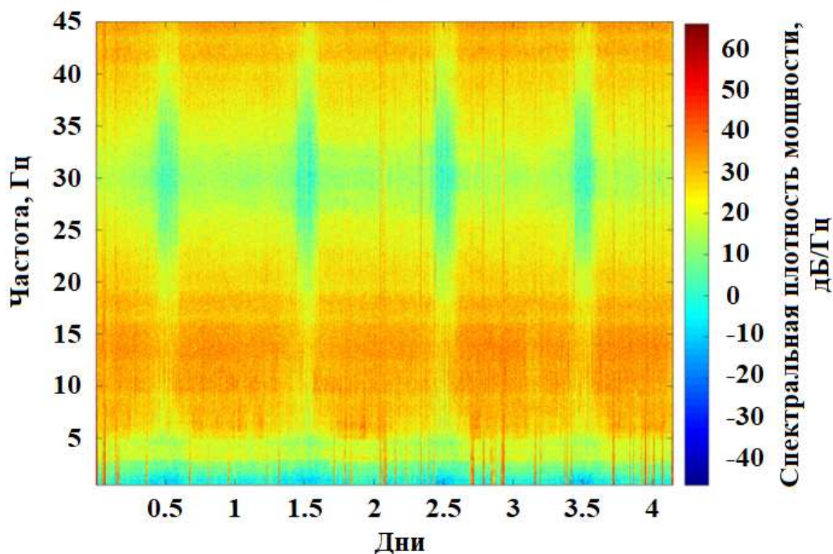
Рис. 18. Спектрограмма вертикальной компоненты колебательной скорости
