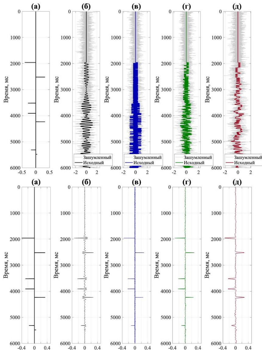
Рисунок 4.2 – Фрагменты сигналов, полученных при моделировании вибрационного зондирования с различными управляющими воздействиями: (а) — импульсная переходная характеристика системы «среда–установка» при x = 0 м; (б) — свип-сигнал с экспоненциальной модуляцией (10–100 Гц), без шума (чёрная) и при \text{SNR} = -2 дБ (серая); (в–д) — сигналы на основе сглаженных ПСП с длительностями 3, 12 и 48 мс (синяя, зелёная, красная кривые — без шума; бледные — с шумом, \text{SNR} = -2 дБ); На нижней панели: сейсмотрассы после
