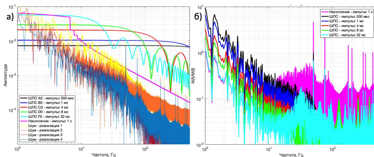
Рисунок 3.4 – (а) амплитудные спектры основных ШПС-сигналов и отдельных реализаций шума; (б) амплитуды отношения спектров шума и ШПС.
