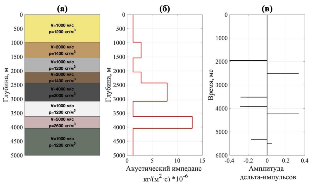
Рисунок 4.1 – Синтетические данные для моделирования сейсмограмм и восстановления ИПХ при различных режимах вибрационного зондирования: (а) многослойная геологическая модель; (б) профиль акустической жёсткости; (в) ИПХ системы "среда–установка" при нулевом расстоянии между источником и приёмником.
