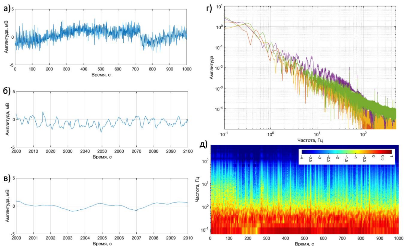
Рисунок 3.2 – Характеристики сигнала-помехи по экспериментальным данным [Кошурников и др., 2024]: (а–в) — фрагменты шума различной длительности; (г) — амплитудные спектры нескольких реализаций шума; (д) — спектрограмма.
