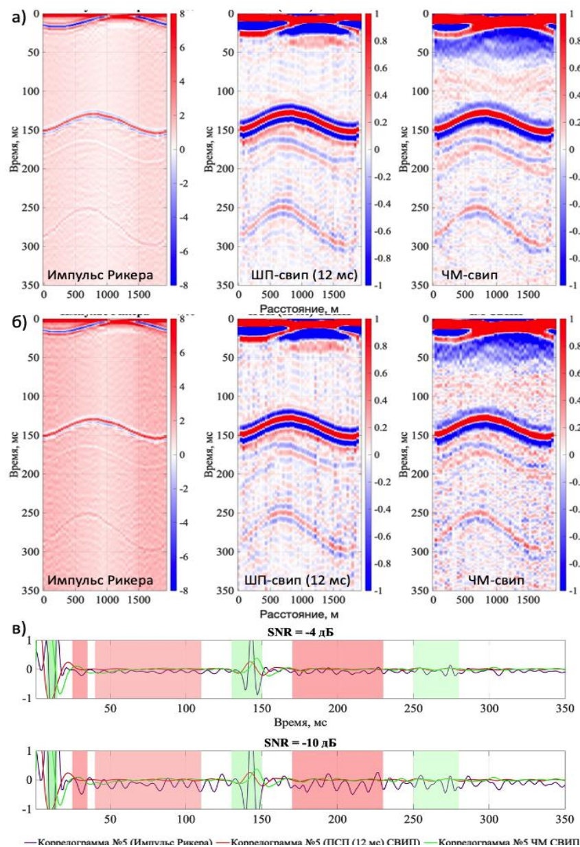
Рисунок 4.4 – Сравнение результатов использования различных управляющих сигналов (импульс Рикера, ШПС-сви́п с длительностью импульса 12 мс, ЧМ-сви́п) в системе вибрационной сейсморазведки малой глубинности: а) сейсмические изображения для трёх рассмотренных управляющих сигналов при отношении сигнал/шум -4 дБ; б) то же при отношении сигнал/шум -10 дБ; в) Примеры нормированных сеймотрасс для одного из каналов.
