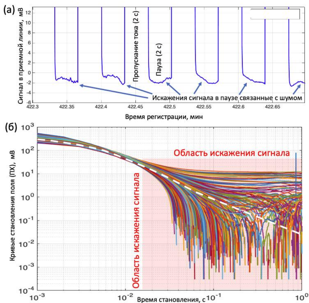
Рисунок 3.1 – Примеры данных ЗСБ, полученных в ходе экспедиции НИС «Академик Мстислав Келдыш», 2020 г. (море Лаптевых). (а) 25-секундный интервал записи; (б) серия кривых становления поля, белый пунктир — синтетическая кривая для обобщённой геоэлектрической модели района.
