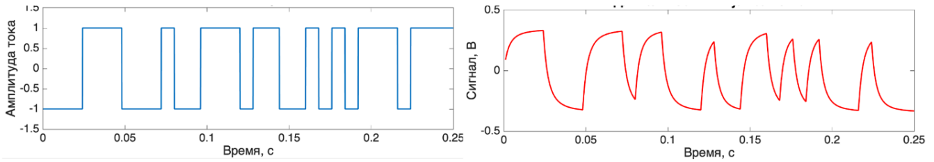
Рисунок 2.1 – Слева: пример сигнала источника с длительностью элементарного импульса (кодového элемента) 8 мс; справа: соответствующий ШПС-отклик.
