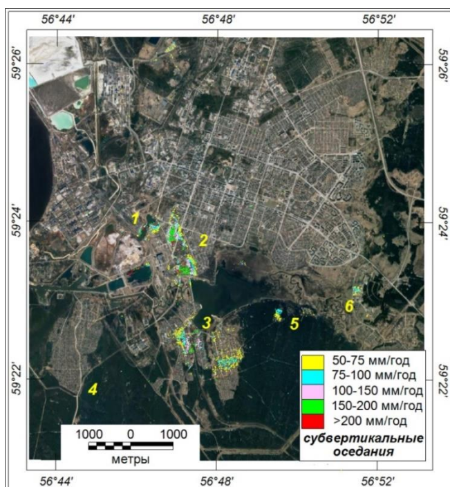
Рисунок 4 – Средние скорости оседаний устойчиво отражающих объектов (в мм/год) для центральной части г. Березники, полученные методом устойчивых отражателей в 2021 г.
